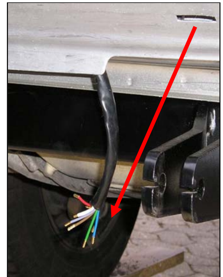
Steckdosenanschlusskabel nach außen führen und danach Steckdose nach Plan anschließen
