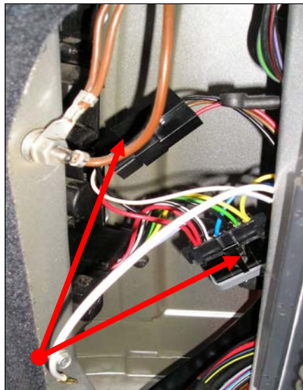
Anschluss Elektrosatz linkes Rücklicht
